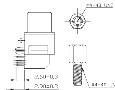
D723X (鉚合附螺絲)
