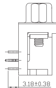
D212X (鉚合鎖螺絲)
