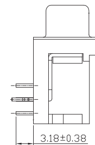
D213X (鉚合附螺絲)
