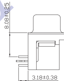
D1110 (鉗合無螺絲)
