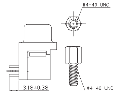
D113X (鉗合附螺絲)
