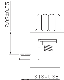
D114X (叉鎖)
