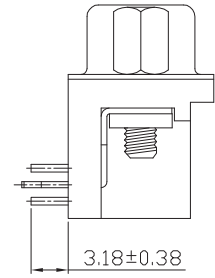
D112X (鉚合鎖螺絲)
