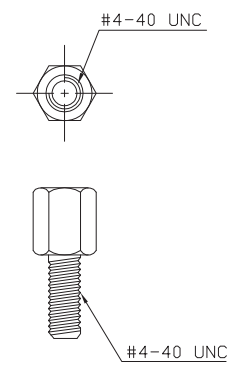
D113X (鉚合附螺絲)
