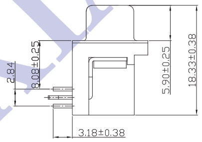
D1110 (鉚合無螺絲)
