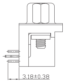
D112X (鉚合鎖螺絲)
