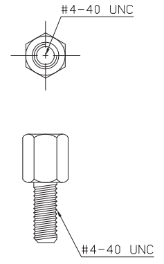
D113X (鉚合附螺絲)
